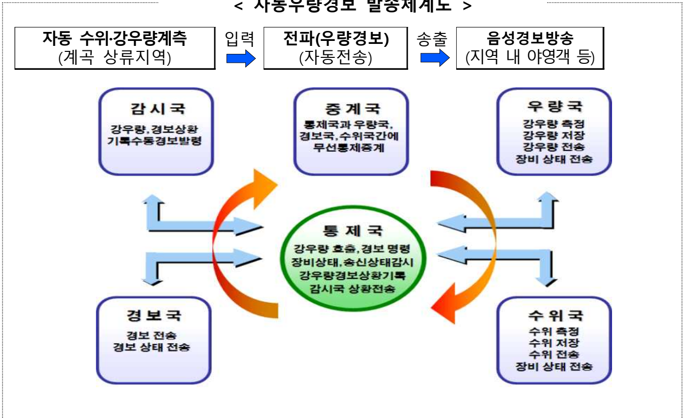
< 자동우량경보 발송체계도 >
